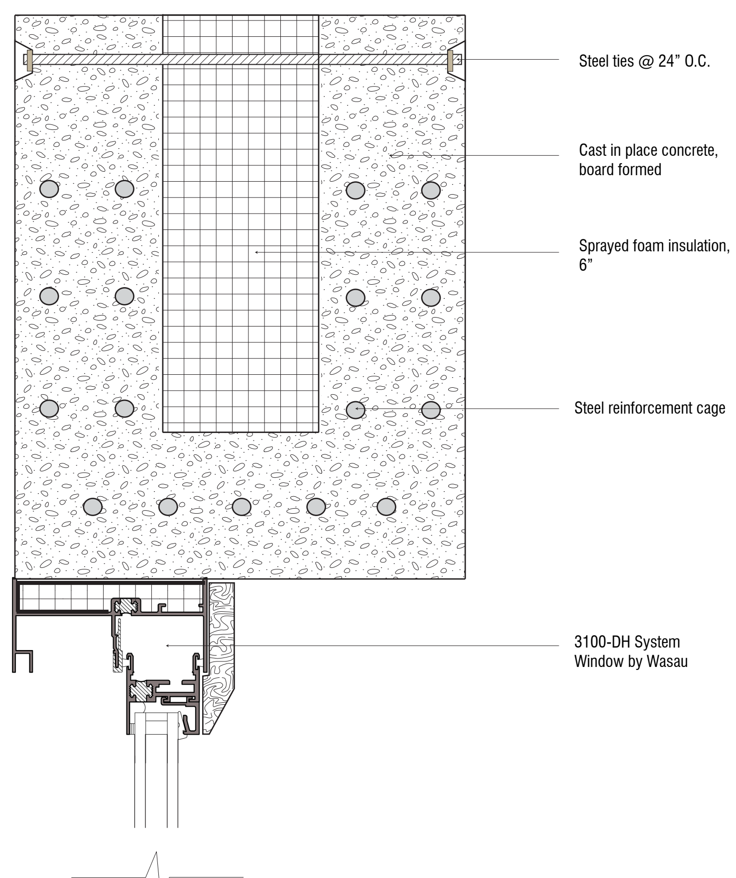
DETAIL // JAMB // 3" = 1'
