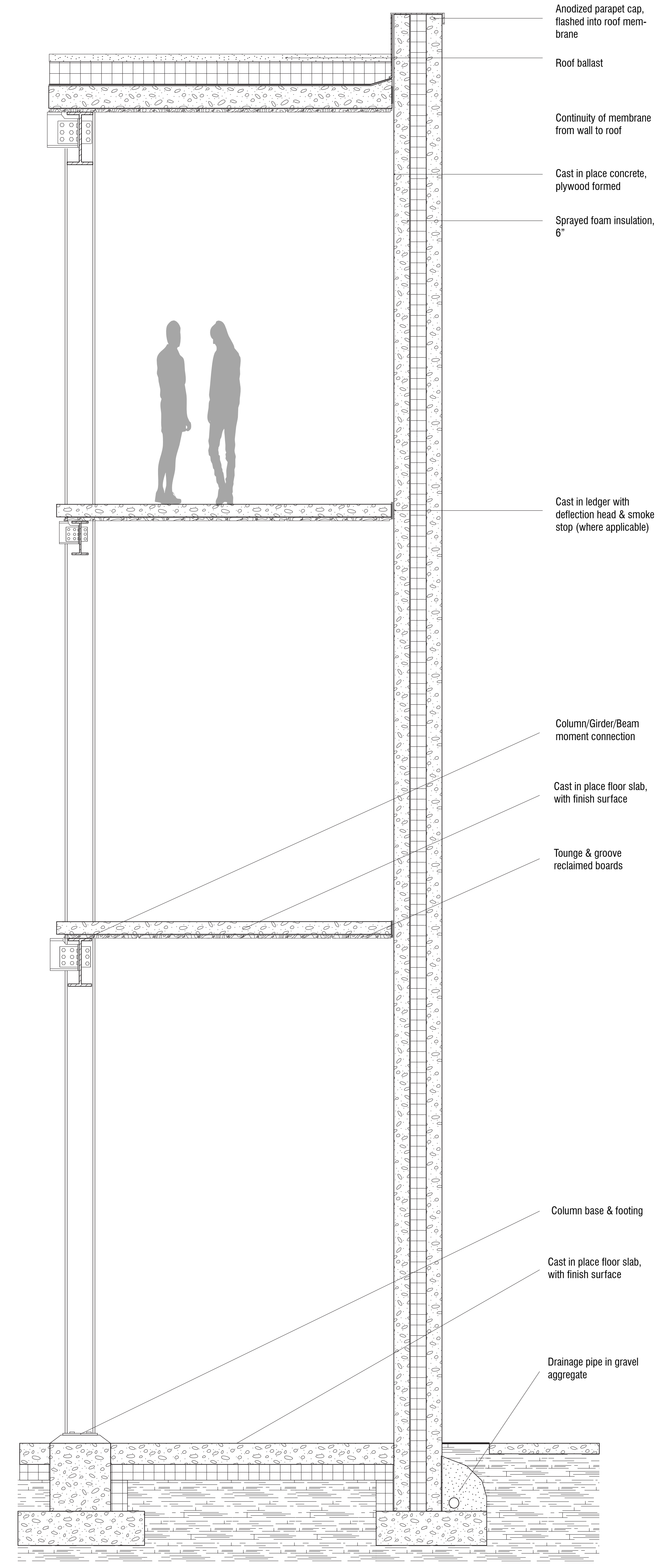
DETAIL // WALL SECTION // 1/2" = 1'
